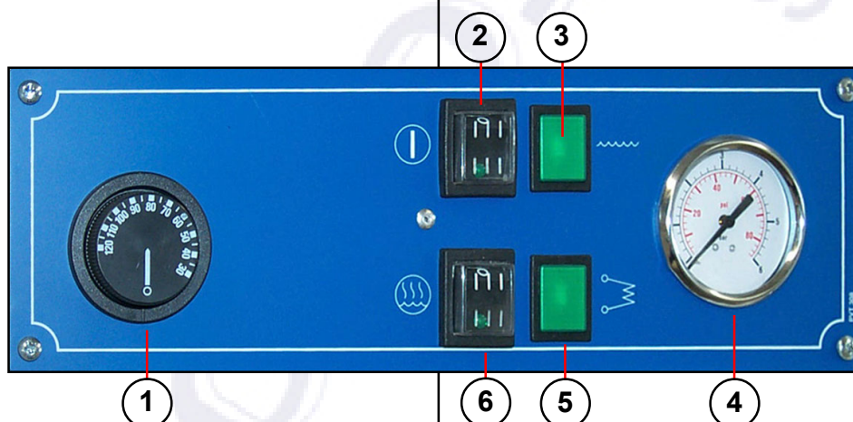
Figura cap. 7.3 "Pannello elettrico Mod. PVT 38 "
